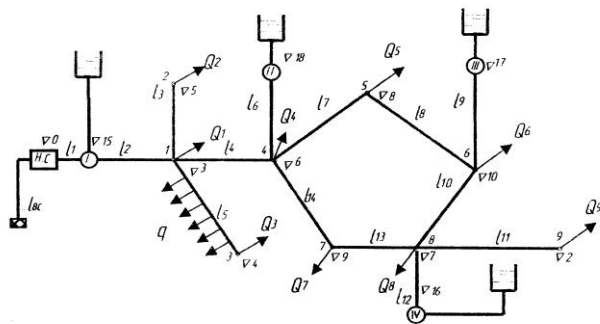
Рис. 1. Общая схема водопроводной сети: I-IV – варианты водонапорных башен; Q – узловые расходы; q – путевой расход; \nabla – отметки поверхности земли в узловых точках
