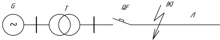
Рис. 1.3. Принципиальная электрическая схема испытания автоматического выключателя
