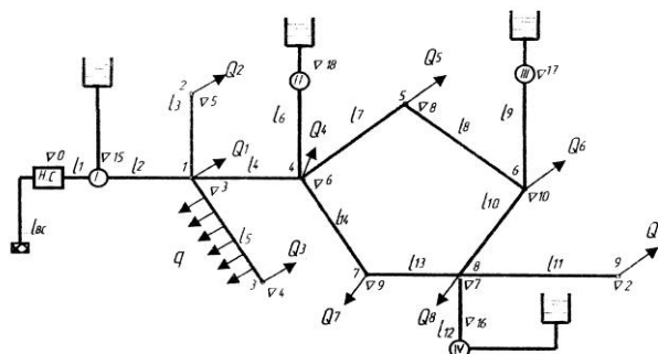
Рис. 1. Общая схема водопроводной сети:
