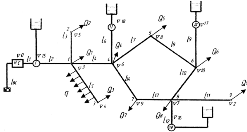
Рис. 1. Общая схема водопроводной сети:
