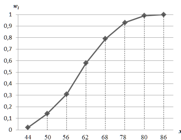
Рис. 1. График эмпирической функции распределения
